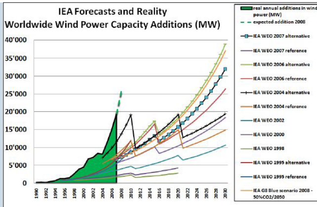
IEA-Wind-Wachstumsprognosen: überholt
